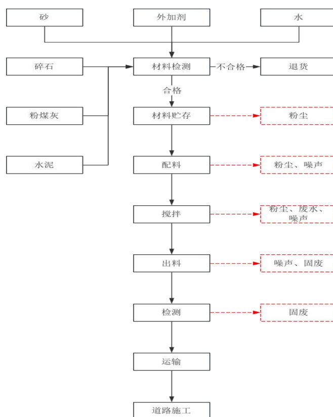
图 2-3 混凝土生产工艺流程图
